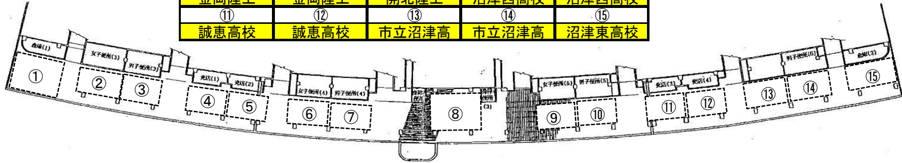
2階天井伏図 1/200
